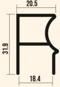
4023 K / MİNİSURF KULP
