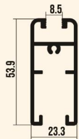
SR 2553 / ALT KAYIT (ÇİFT TEKER)
