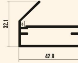
7925 FK / YAPIŞMA ÇERÇEVE KULP
