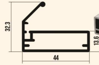
7909 FK / BOY KULP
