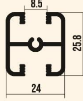
SR 2126 / ORTA ÇİTA
