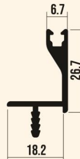
4050 MK / CUMBA KULP
