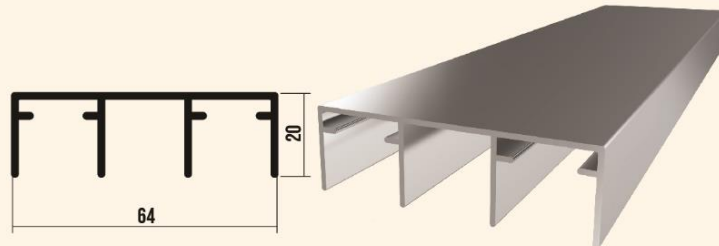
3080 R / SKM80 ÜST RAY
