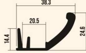
7302 FK / FİX ÇERÇEVE KULP
