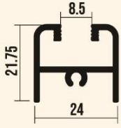
SR 2122 / ÜST ÇİTA
