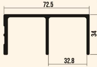
SR 2472 / GAMA ÜST RAY
