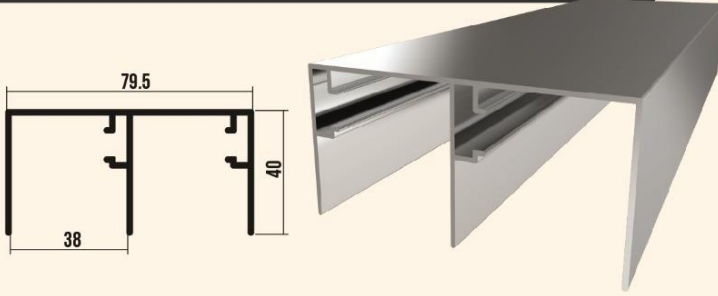
3100 R / SRG100 ÜST RAY
