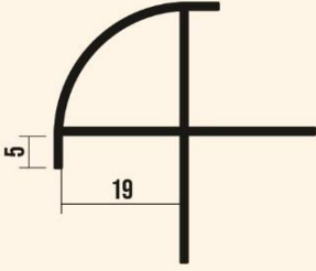
5712 S / KÖŞE DÖNÜŞ
