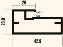
7046 F / 20X42 ÇERÇEVE
