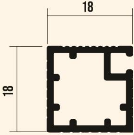
6250 M / EVYE KAYIT
