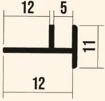
5106 S / CAM ÇITASI
