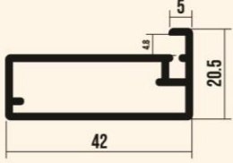
7301 F / FİX ÇERÇEVE
